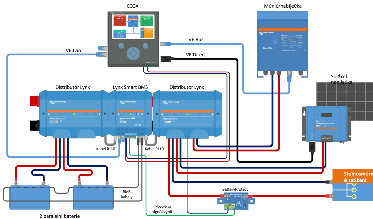
Systém s lithiovými bateriemi, Lynx Smart BMS a dvěma Lynx Distributory
